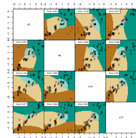
Fehlerraten bei 2-Organ-Kombinationen
