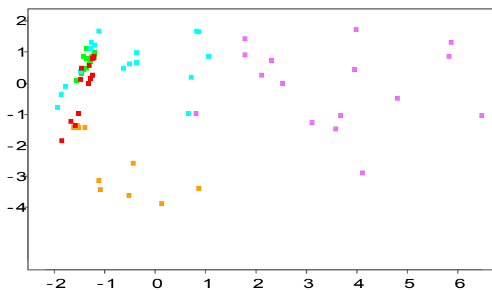
Trennung der Therapieklassen mit 2 Diskriminanzkomponenten aus 6 Organen
