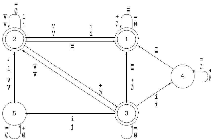
Abbildung 4.2: Endlicher Automat für die Plural-i-Regel
