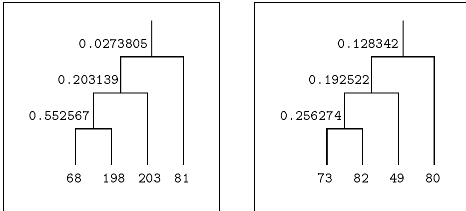
Abbildung 5.1: Ausschnitte aus der Clusterhierarchie vom 23.01.97
