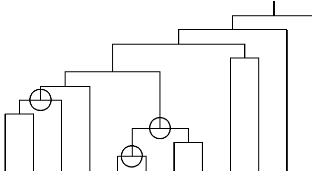
Abbildung 4.4: Dendrogramm
