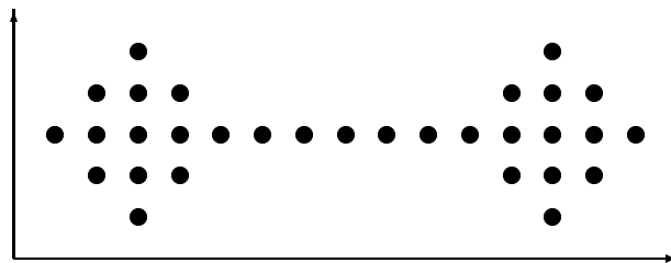
Abbildung 4.5: Chaining
